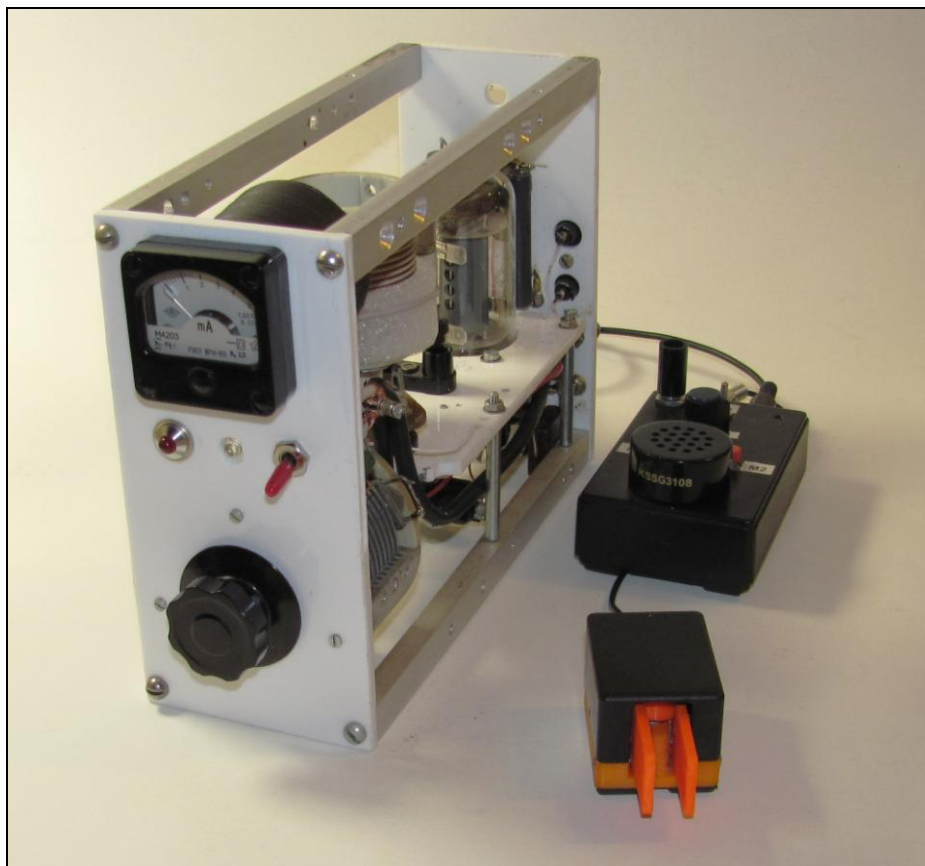
Vysílač pro QRP MAS Contest, viz str. 29
